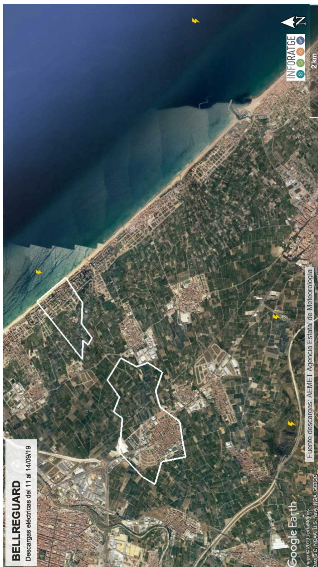
Geolocalización de las descargas eléctricas ⁂ nube-tierra ⁂ registradas en el término municipal de BELLREGUARD y alrededores entre el 11 y el 14/09/19 Fuente descargas: AEMET Agencia Estatal de Meteorología
