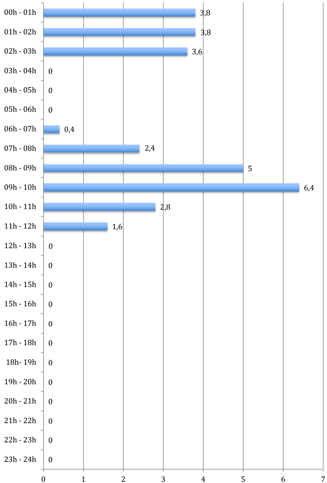
Cantidades de lluvia registradas por horas en BELLREGUARD el día 12/09/19 (en l/m²)
